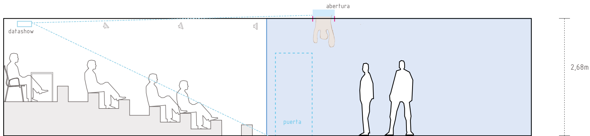
corte lateral
